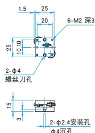
AIS-25B 圆头小螺栓 M2×6...2个, 平垫圈
