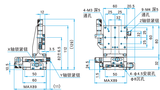
TSDS-605SL 内六角螺栓 (不锈钢) M4×6...4个
