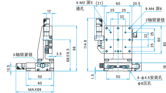
TSDS-604SL 内六角螺栓 (不锈钢) M4×6...4个
