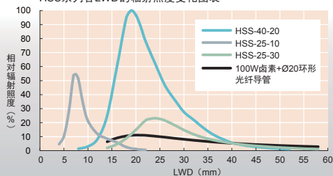
HSS系列各LWD的辐射照度变化图表
