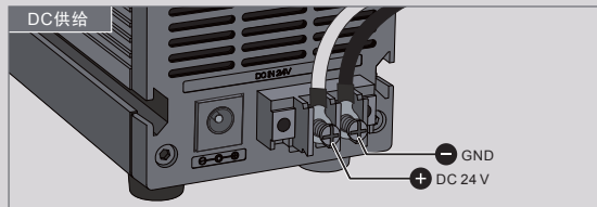
DC24V输入使用主体背面的端子排。
