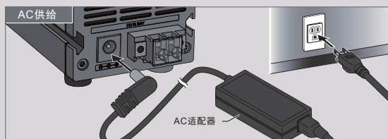
AC100-240V输入需使用AC适配器（选件）。 型号：A-P2460-PFB-JTLV6（遵从美国DoE CEC Level VI外置电源规定）
