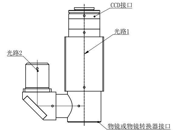
比例: 1:2 光路1: 0.5倍成像光路 光路2: 照明光路
