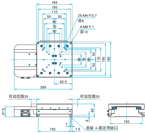
HST(GS)-50X-0B 内六角螺栓 M6×15...4个
