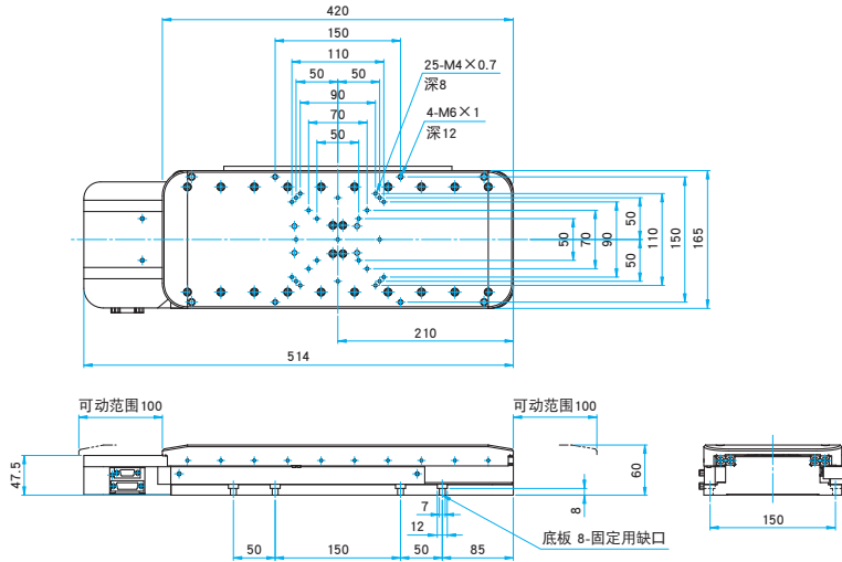
HST(GS)-200X-0B 内六角螺栓 M6×15...8个
