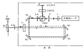
图 1 光学系
