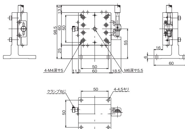
↑ LZ-6047-S6
