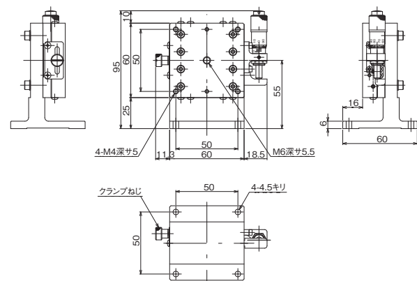
↑ LZ-6047-S8
