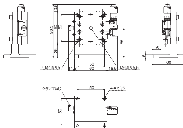
↑ LZ-6047-S1
