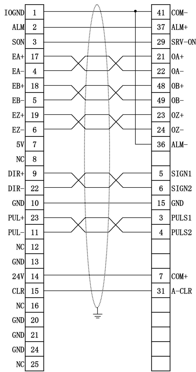
控制卡NMC3400 Panasonic MSDA系列 AXIS1-AXIS4 驱动器接口
